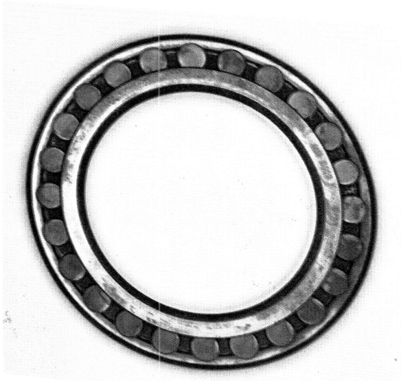
Bild F 44 Havarie spuren — Lauf- farbe nach "am Wälz " lager einem Brand
