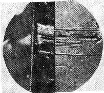
Bild 111 Vergleich einer Werkzeugspur
