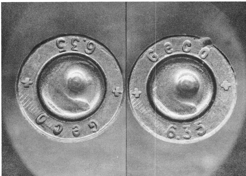
Bild 98 Schußwaffenidentifizierung — Gegenüberstellung von Tat- und Vergleichshülse
