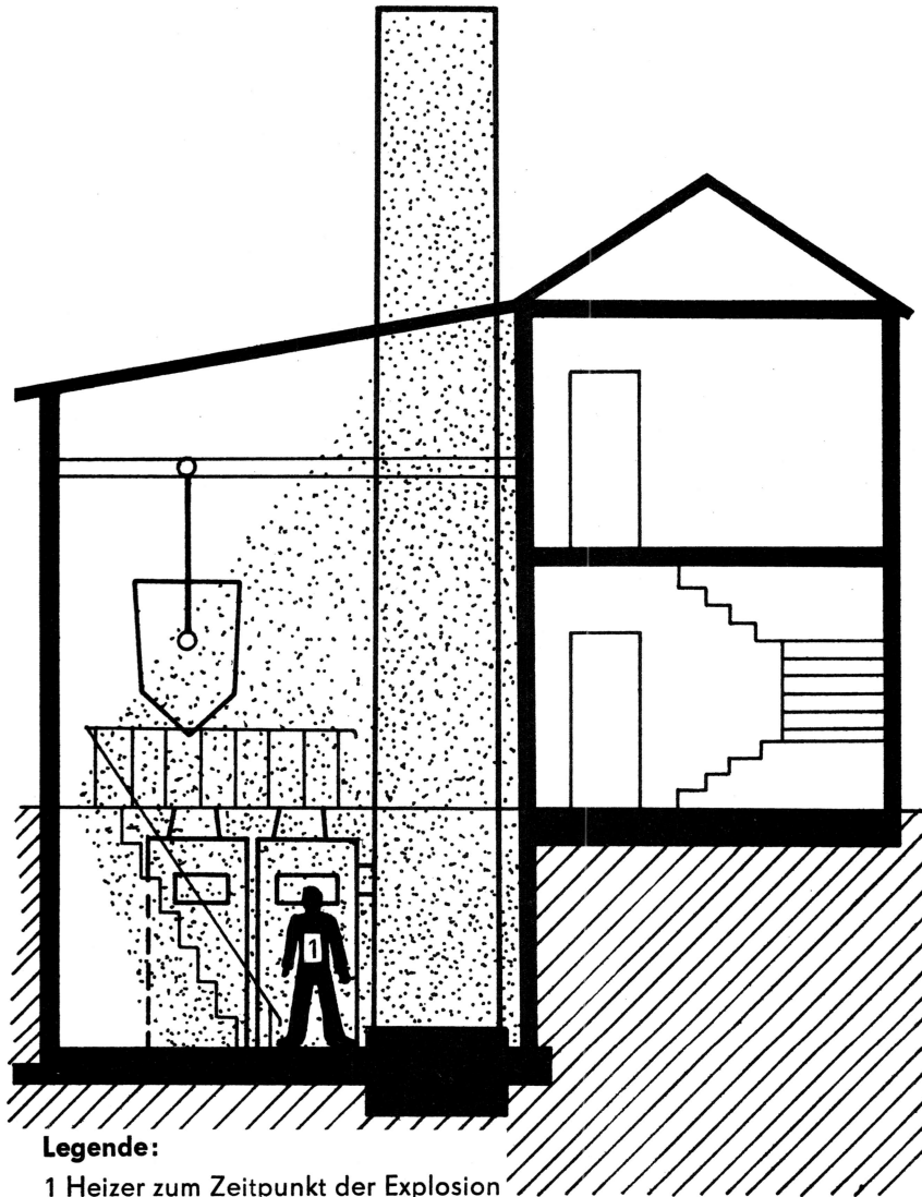
Bild 93 Schnittzeichnung
