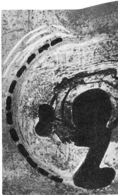
Bild 91 Spuren eines schloßfremden Werkzeugs an dem Schloßriegel
