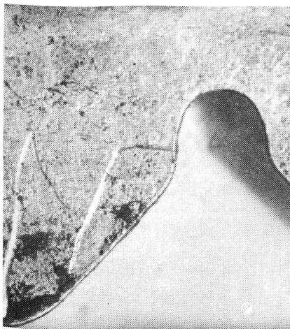
Bild 91 Spuren eines schloßfremden Werkzeugs an dem Schloßriegel
