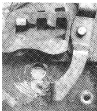
Bild 92 Schlüsselspuren auf dem Boden eines Chubbsschlusses
