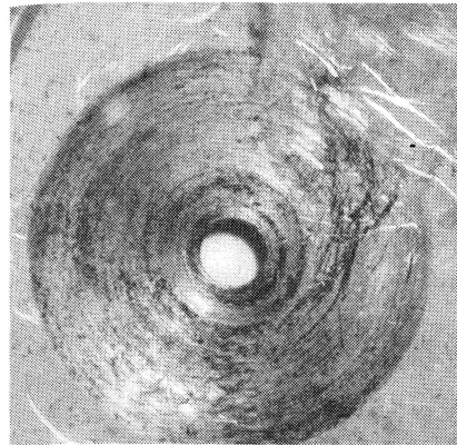
Bild 90 Durch Sperrhaken verursachte Schartenspur und Kratzer außerhalb des Schlüsselbartradius auf dem Schloßboden
