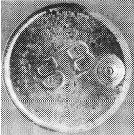
Bild 85 Schlagbolzenspur bei Randfeuerzündung
