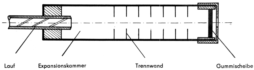
Bild 84 Schematische Darstellung eines Schalldämpfers
