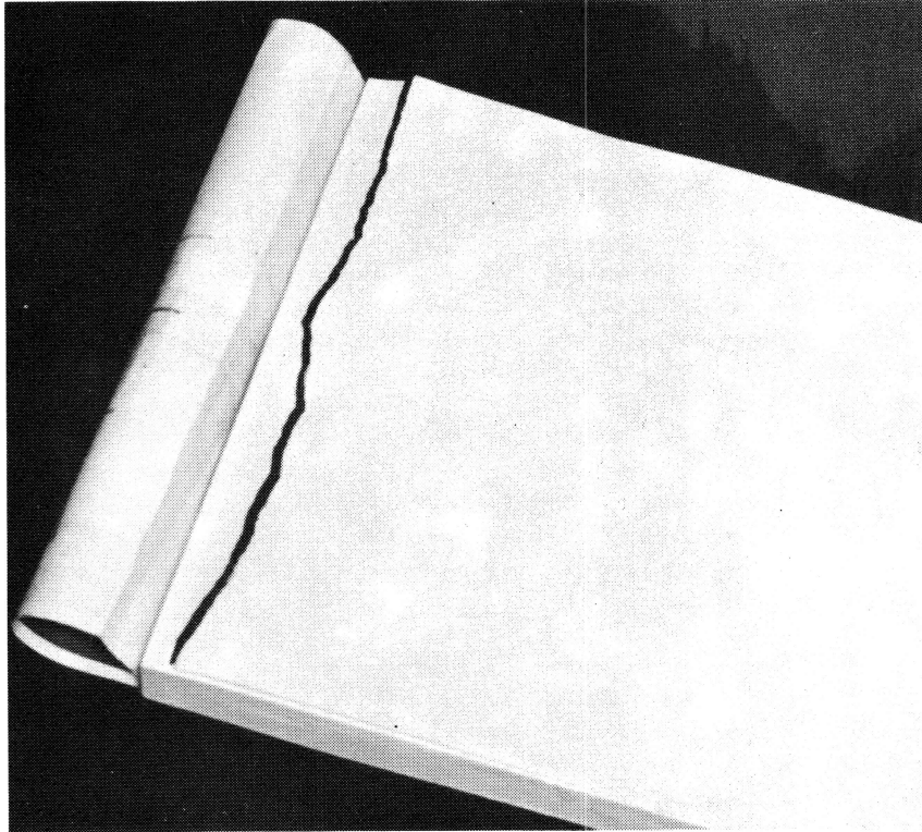
Bild 83 Rißkantenvergleich
