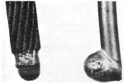
Bild 53 Kurzschlußtypische Schmelzperlen an Kupferleitung
