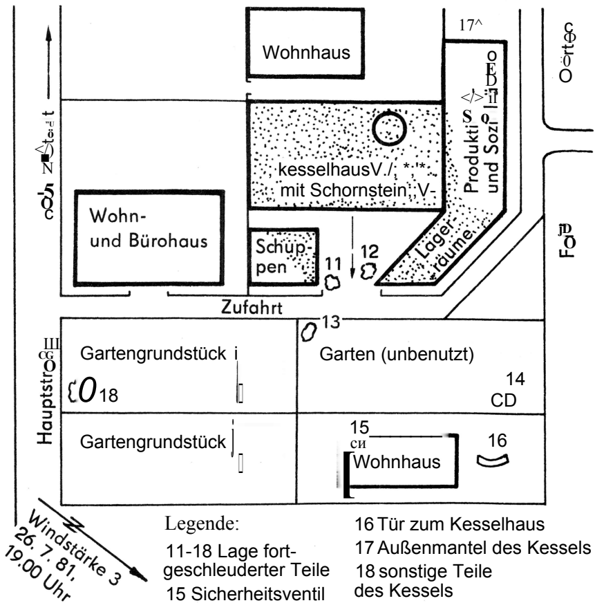
Bild 54 Lageplan
