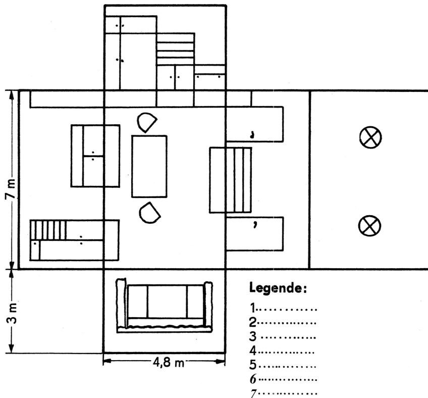
Bild 52 Kreuzprojektion
