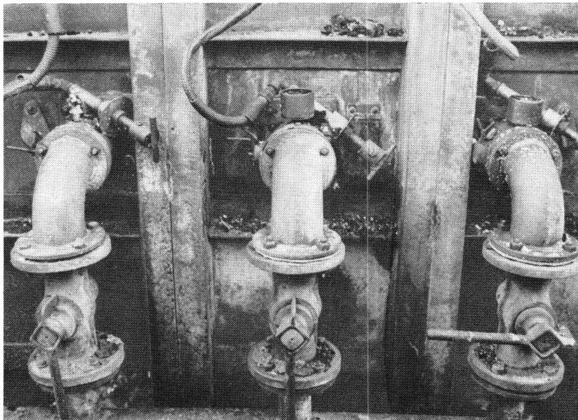
Bild 45 Havarie spur — Schaltstellung von Einwege-Hähnen in Rohrleitungen
