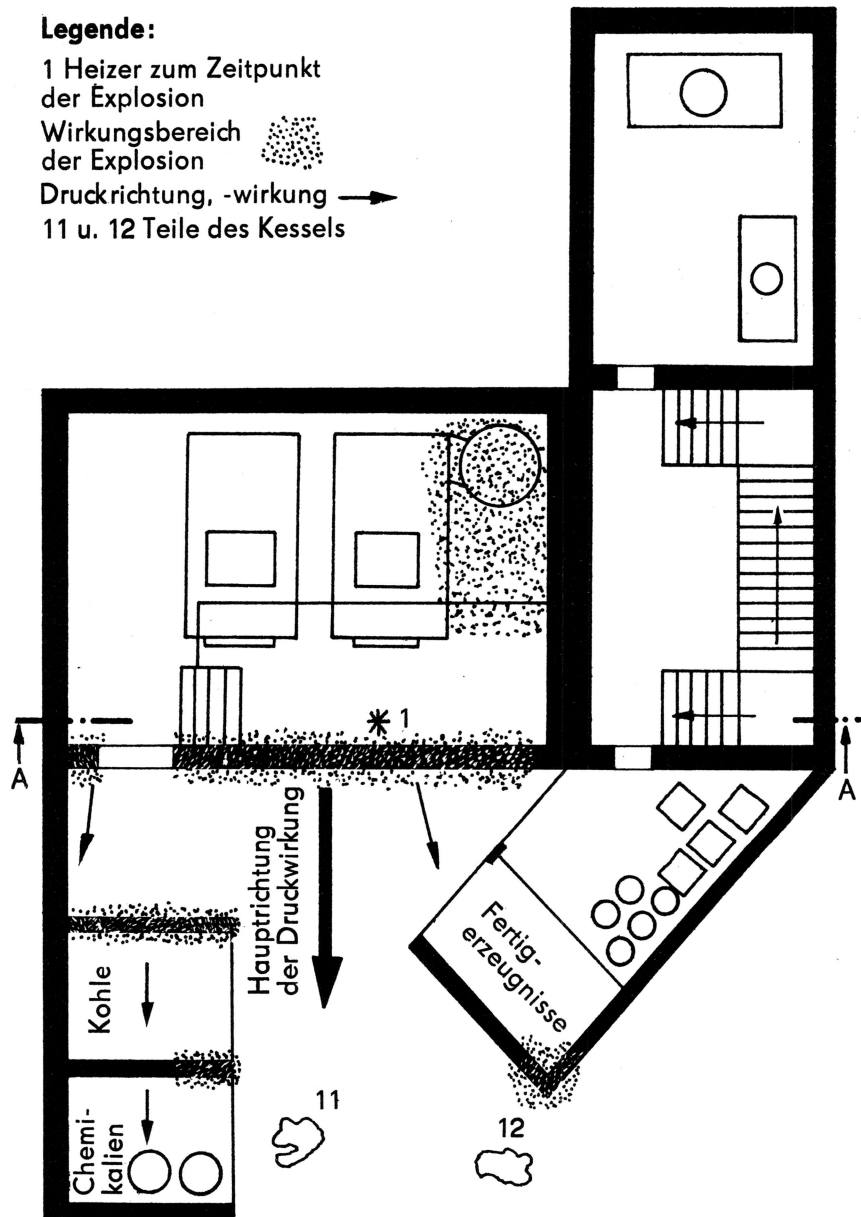
Bild 43 Grundrißzeichnung
