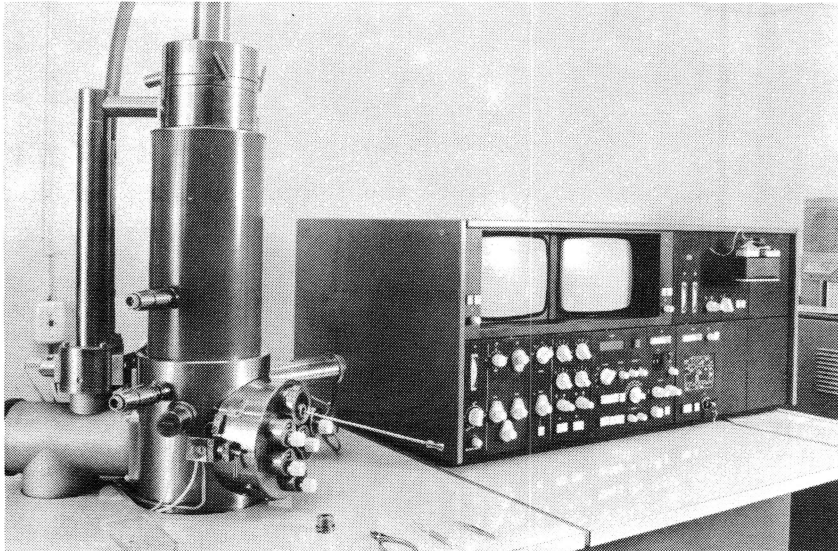
Bild 32 Rasterelektronenmikroskop BS 300
