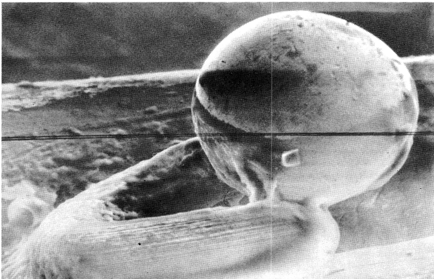
Bild 33 Rasterelektronenoptisches Bild eines Glühlampenwendels — mit Schmelzperle
