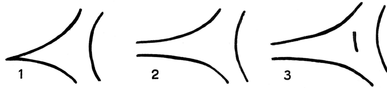
Bild 26 Deltaformen 1 _ geschlossenes Delta, 2 — offenes Delta, 3 — offenes Delta mit Einlagerung
