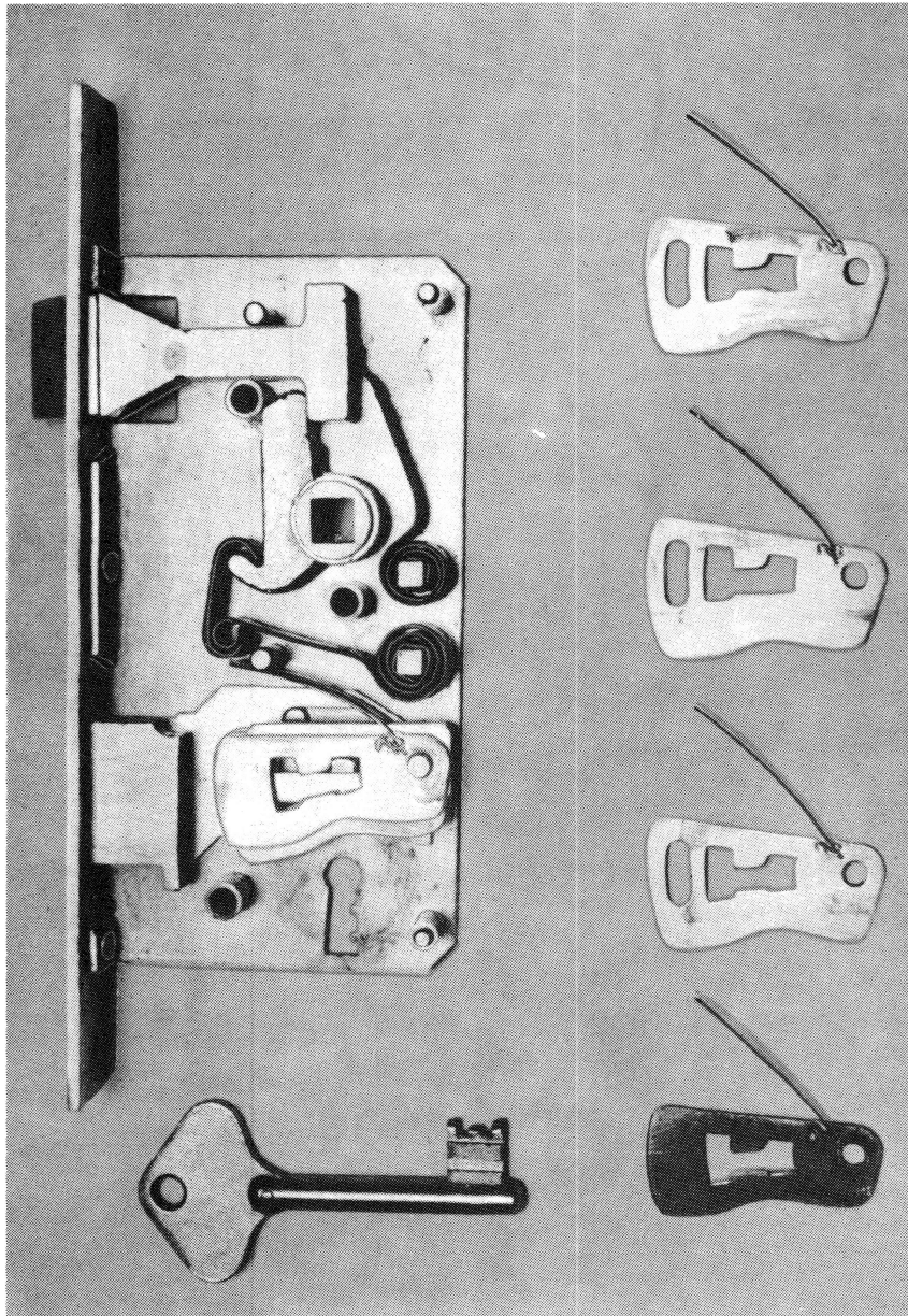
Bild 25 Chubbschloß mit demontierten Zuhaltungen
