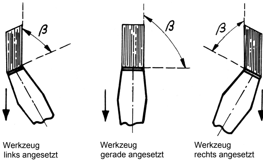
Bild 7 Werkzeugansatzwinkel
