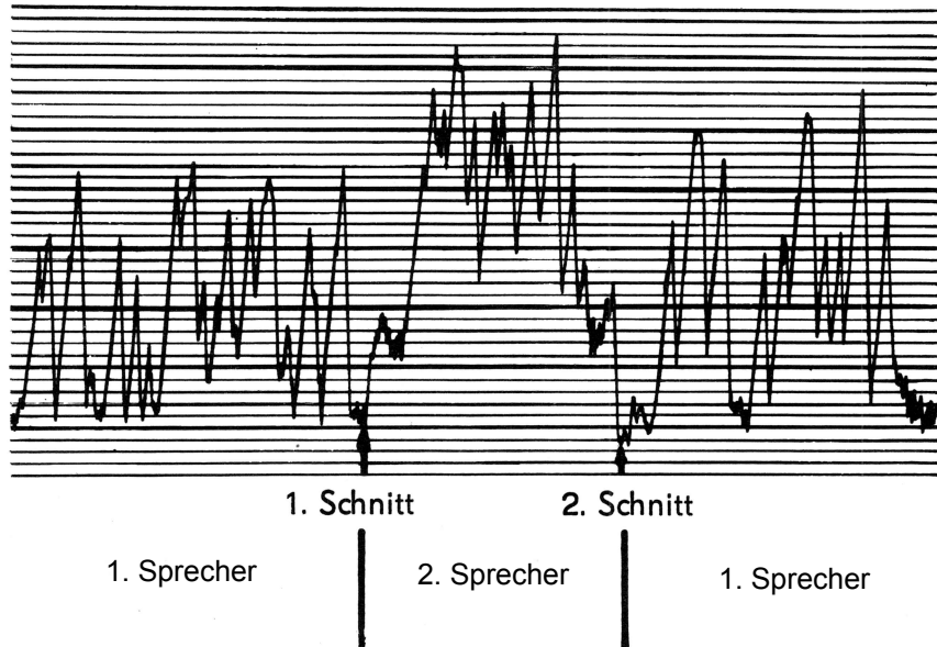
Bild 4 Pegeldarstellung von Sprachmodulationen (Löscheinfügung)
