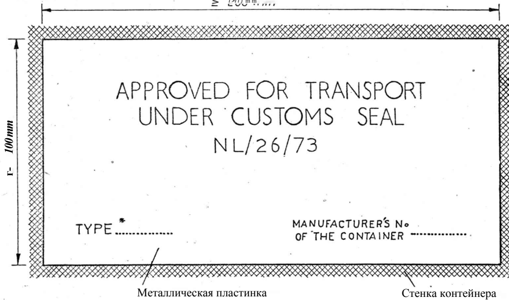
Добавление 1 к Приложению 5 ОБРАЗЕЦ № I ТАБЛИЧКА О ДОПУЩЕНИИ (английский вариант) \geq 200 \text{ mm}
