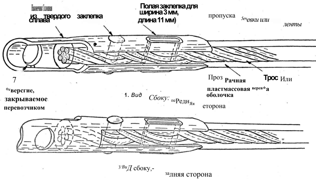
Приложение 4 — Рис. № 5 ОБРАЗЕЦ НАКОНЕЧНИКА
