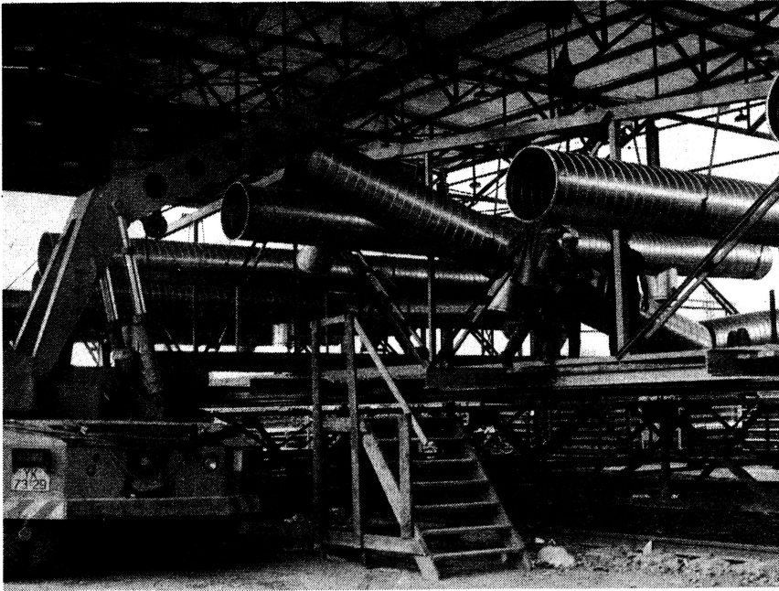
Konsequente Industrialisierung auf der Basis des leichten, ökonomischen Bauens. Unser Bild: Fließbandmäßige Vollmontage von Metalleichtbau-dachsegmenten auf der Baustelle.
