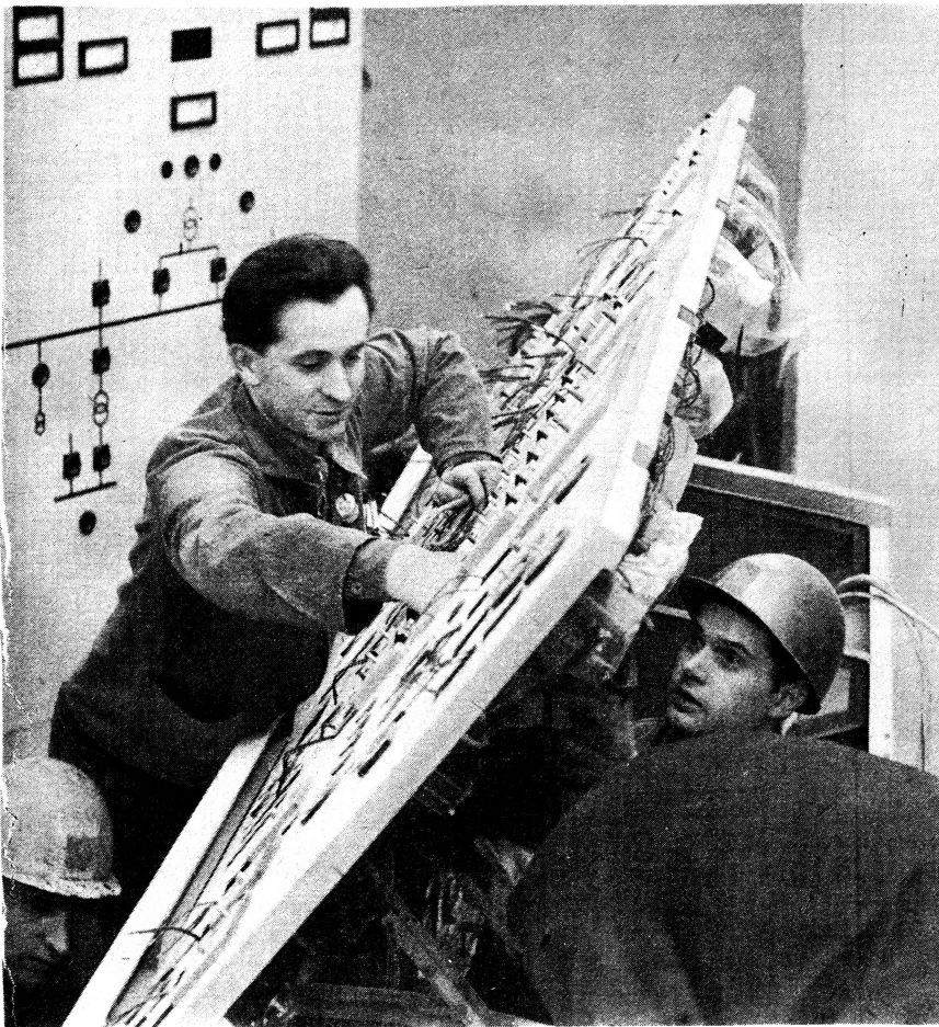
Brigade Romberg beim Installieren der Blockwarte 8 im Kraftwerk Vetschau. Ein Verbesserungsvorschlag des Brigadiers (links oben) bringt einen Jahresnutzen von 180 000 MDN«
