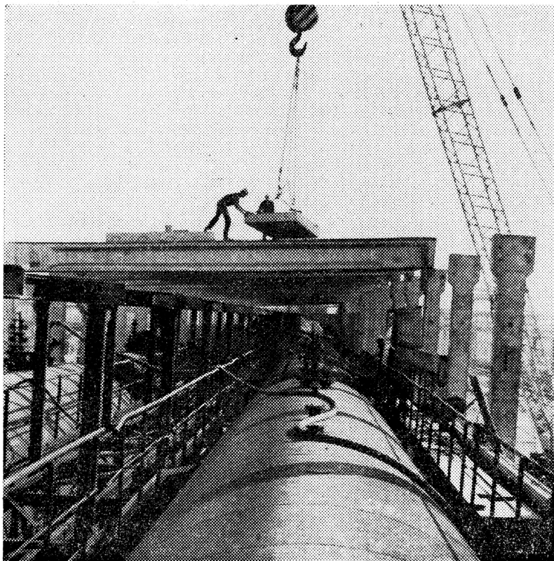
Monteure des Bau- und Mon- tagekombinats Chemie Halle beim Aufbau der Oleum-Anlage der Caprolactam- Fabrik in Leuna II
