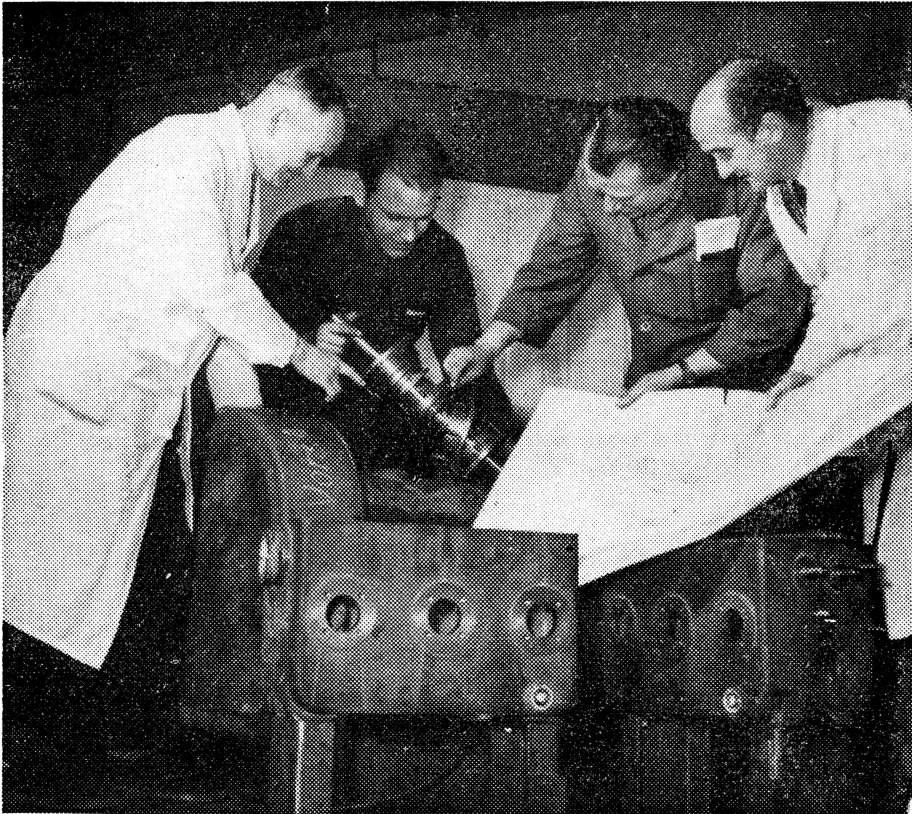
Im VEB Webstuhlbau in Karl-Marx-Stadt entwickelt eine sozialistische Arbeitsgemeinschaft einen Wollwebautomaten mit einer hohen Arbeitsproduktivität. Der Aufbau des Automaten erfolgt nach dem Baukastensystem
