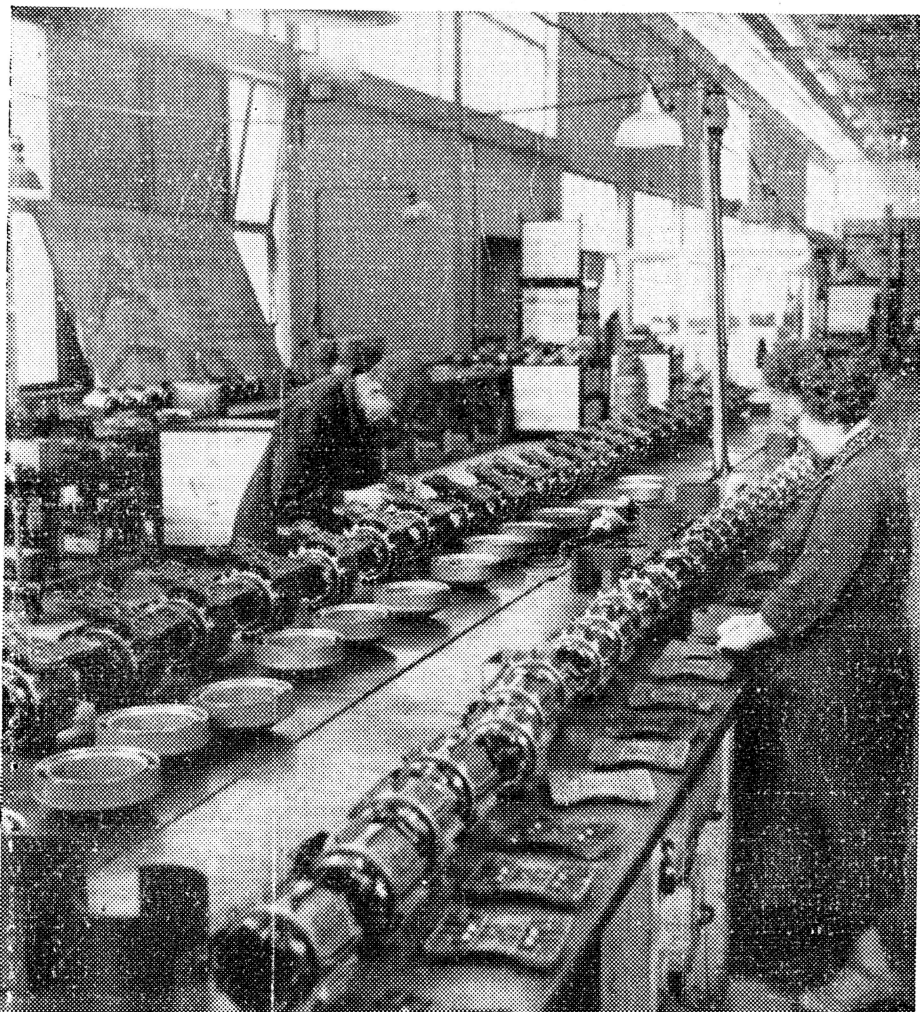
Als Beitrag zur Verwirklichung der Beschlüsse des 8. Plenums verpflichteten sich die Werkötigen der Einheitsmotorenfabrik des VEB Sachsenwerk in Dresden-Niedersedlitz, über ihren Plan hinaus täglich einen Einheitsmotor für die Landwirtschaft zusätzlich zu produzieren. Auf dem Bild die Montiererin Elfriede Engelmann und der Monteur Horst Fellendorf beim Anschrauben der FüÙe an die Motoren
