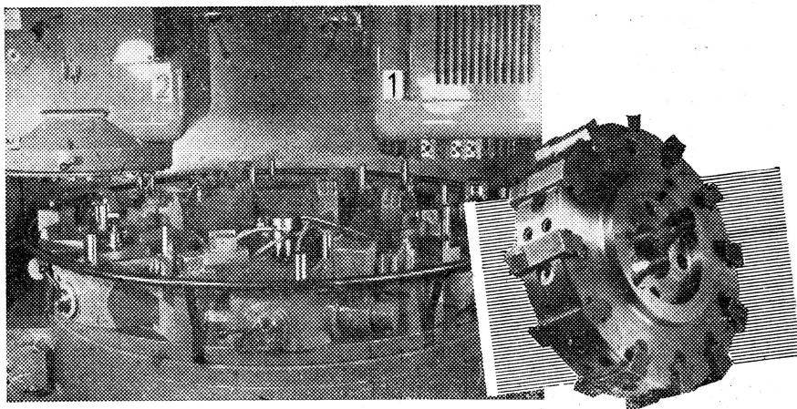
Die Einstell-Messerköpfe vom VEB Werkzeugfabrik Altenburg zeichnen sich durch hohe Spanneleistungen sowie geringen Werkzeug verschleiß aus. Sie helfen Rüstzeiten und Instandhaltungskosten einzusparen. Sie beweisen auf Fräswerken, Taktstraßen und Sondermaschinen ihre hohe Leistungsfähigkeit. Schnelles „Auswechseln“ der Messer durch Exzenterspannung und leichtes Einstellen in radialer und axialer Richtung bis zu 0,015 mm Genauigkeit sind die markantesten Merkmale dieser Neukonstruktion.
