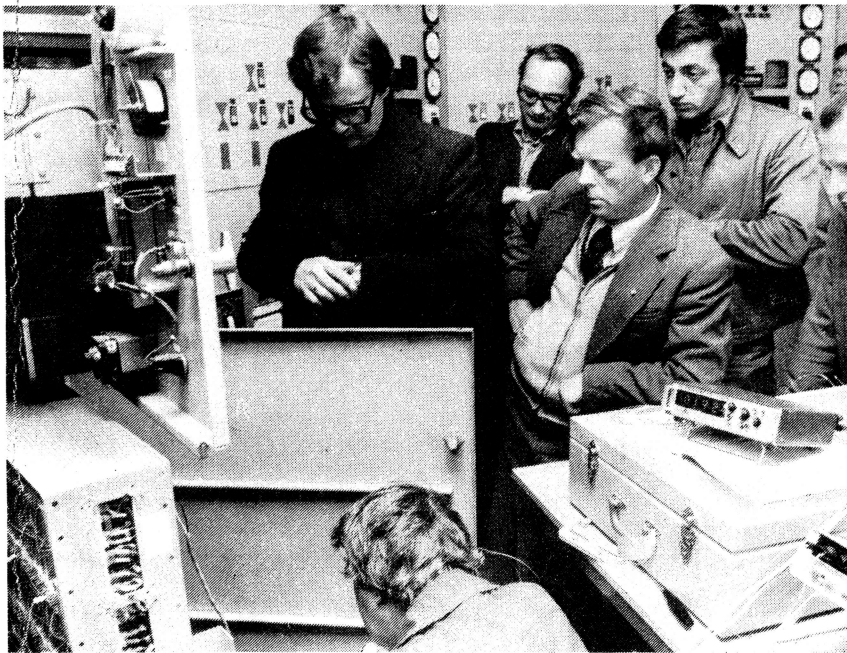
Die erste Verdichterstation der transkontinentalen Erdgasleitung Sojus wurde am DDR-Standort in Talnoje in Betrieb gesetzt. Spezialisten von „Orgenergogas“ aus der UdSSR und DDR-Monteur starteten gemeinsam die erste 10-MW-Gasturbine. Am 26. 9. 1978 wurden alle sieben Verdichter der Station von der staatlichen Kommission mit „Ausgezeichnet“ abgenommen. Foto: ADN-ZB/Busch
